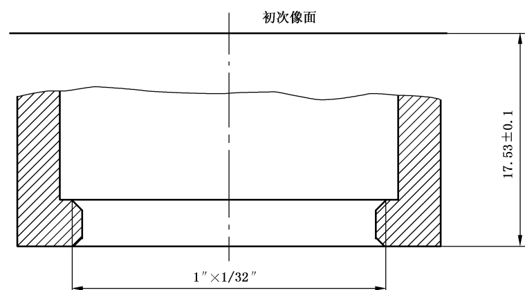
图 2 配合装置尺寸和初次像面的位置
